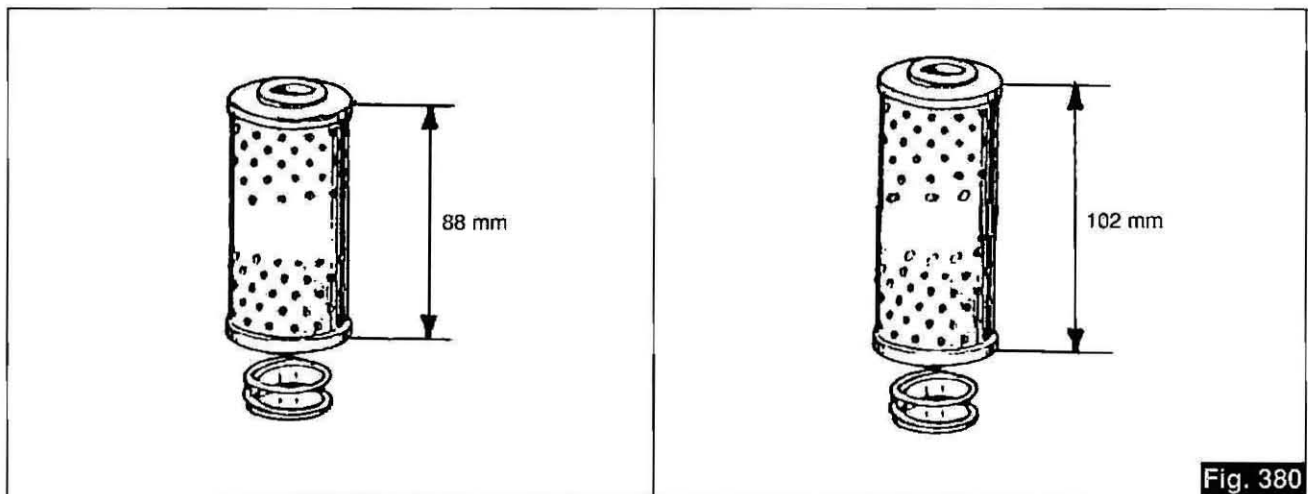
Filtro olio "Basso" cod. 19 15 30 00
