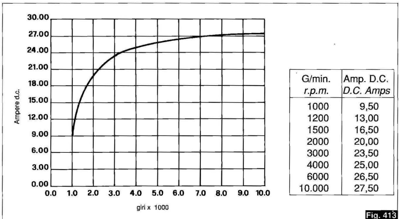
Grafico intensità corrente di carica
