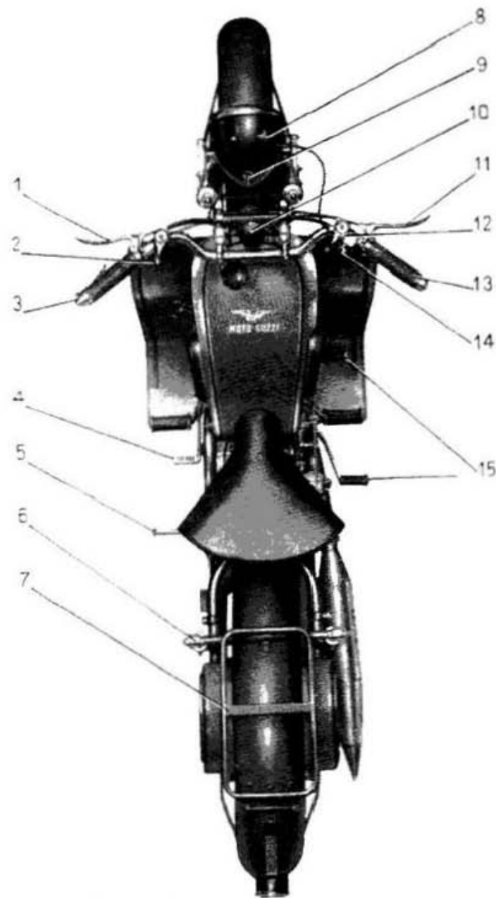
Fig. 3 - Motociclo Astore (comandi ed accessori)
